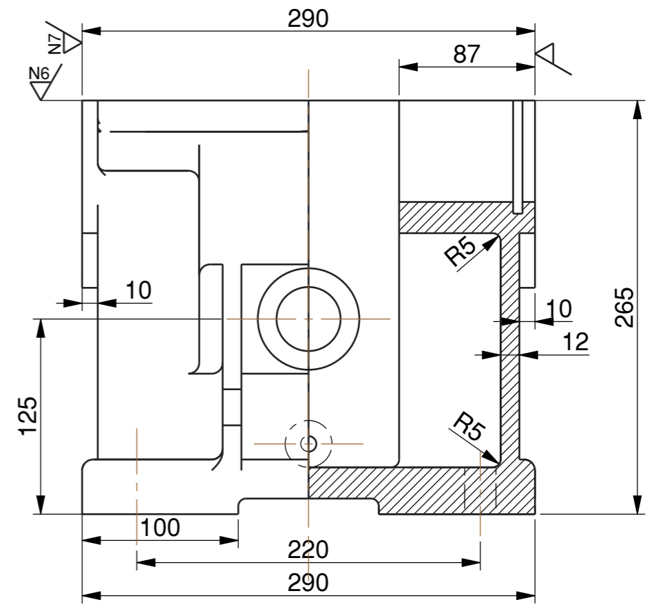
PRESEK A-A
