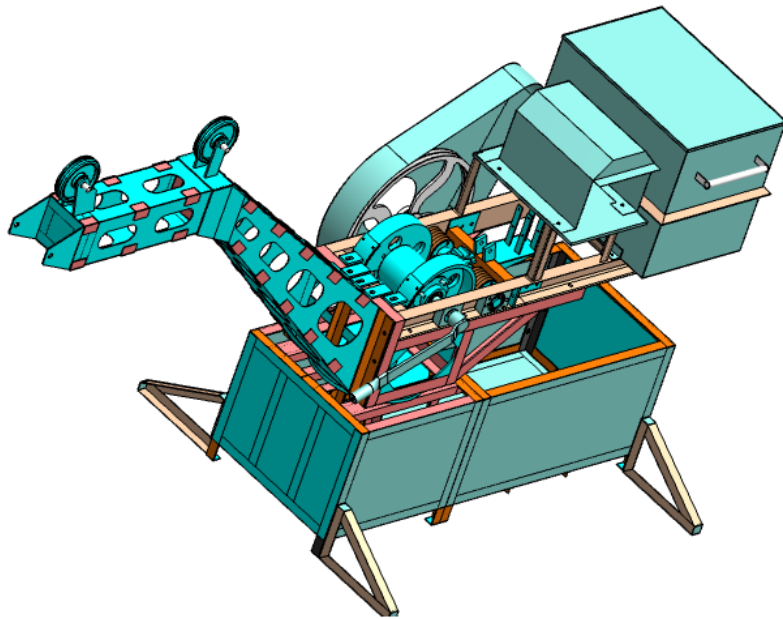
Mini Crane
