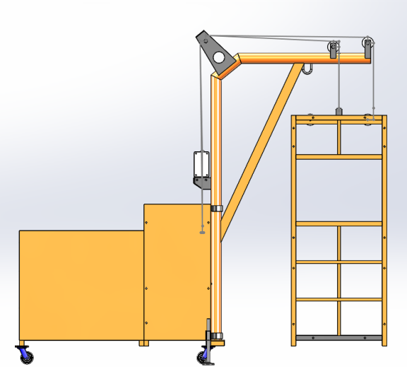
Mini Lift
