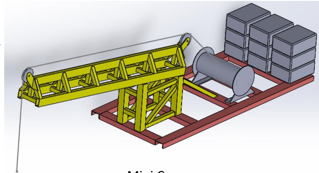
Mini Crane
