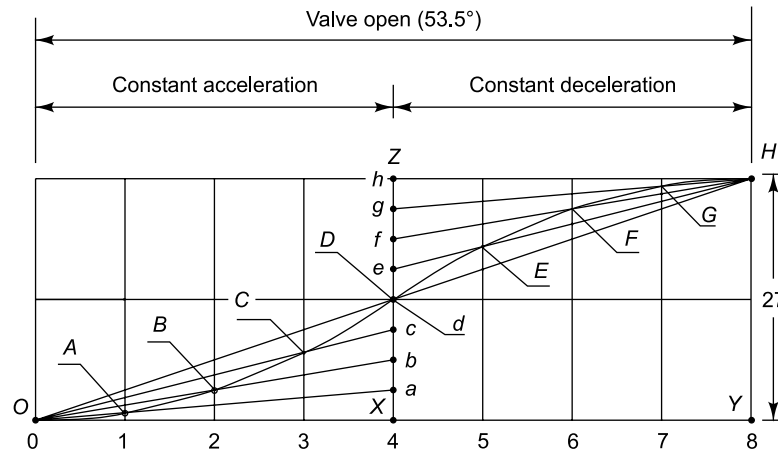
Fig. 25.44 Displacement Diagram
