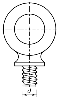
Fig. 7.13 Eye Bolt
