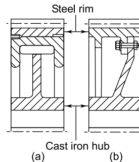
Fig. 17.36 Rimmed Gears
