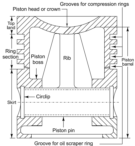
Fig. 25.4 Piston
