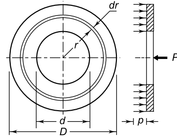
Fig. 11.3 Friction Disk
