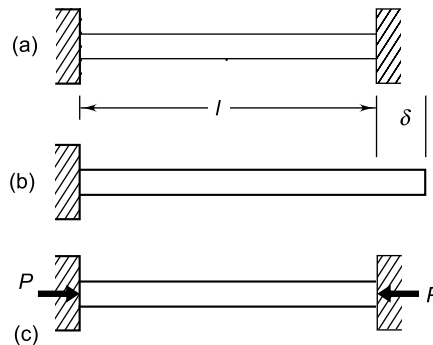
Fig. 4.69 Thermal Stresses
