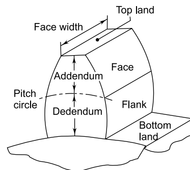
Fig. 17.7 Gear Nomenclature
